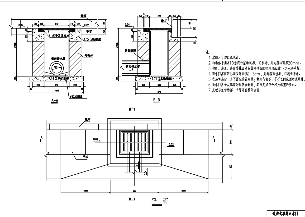
边沟式单篦雨水口
